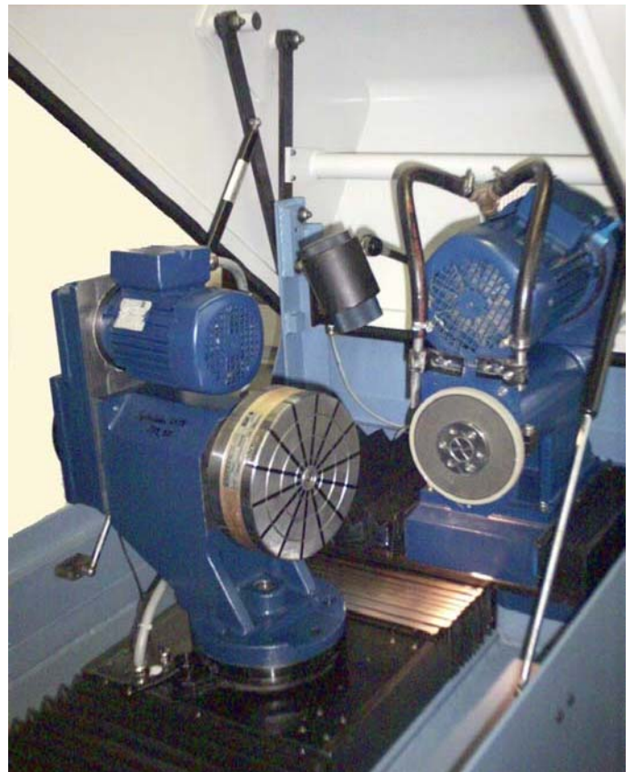
Flexible Werkstückaufnahme mit Magnetspannplatte (wahlweise) und Encoder
